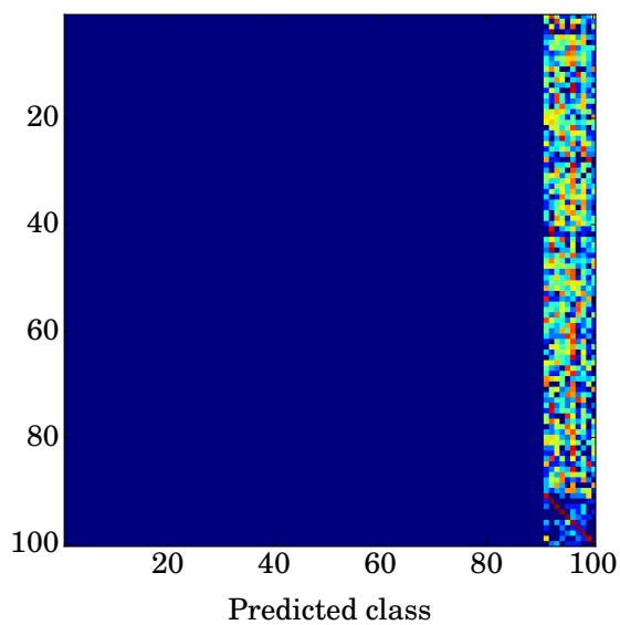
(d) finetuning
